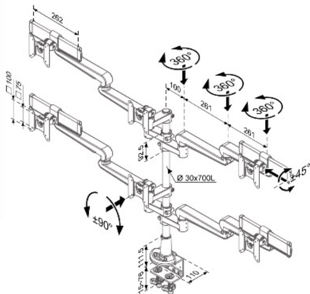
Clamp Type unit:mm
